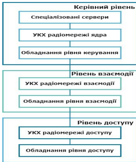
Рис. 5. Узагальнена структура мережі зв'язку АСУ низової ланки управління
